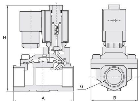
Рисунок 1. Эскиз
